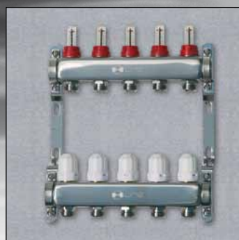
Art. H-LINE 1175.xxx rozdělovač pro podlahové vytápění s průtokoměry - přívod G1/2" - připojení okruhů G3/4"x18 EUROCONUS
