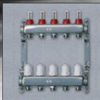
Art. H-LINE 1175.xxx rozdělovač pro podlahové vytápění s průtokoměry - přívod G1" - připojení okruhů G3/4"x18 EUROCONUS
