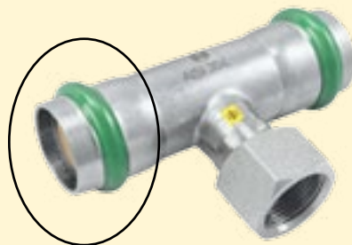
indikace nezalisovaného spoje
