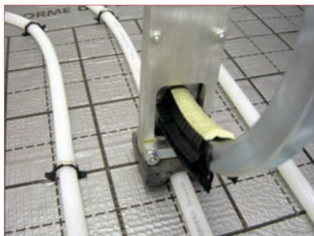
upevnění trubky k izolační desce pomocí úchytů
