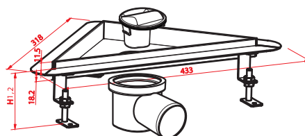
art. PB.SYK0301 rohový odtok ke zdi
