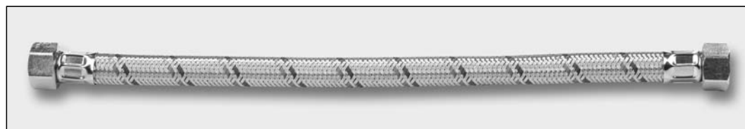
Art. INOX 100 - 160 nerezové opletené hadičky s int. těsněním, EPDM 9 x 13 mm, PN 10, T = 90°C
